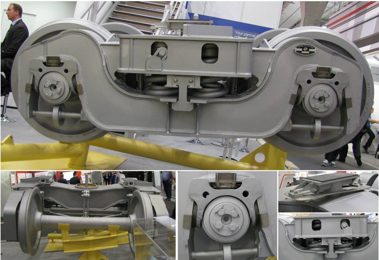
Güterwagen-Drehgestell/Freight Car Bogie TTV T 25 (für 1524 mm Breitspur/1524 mm Gauge)
