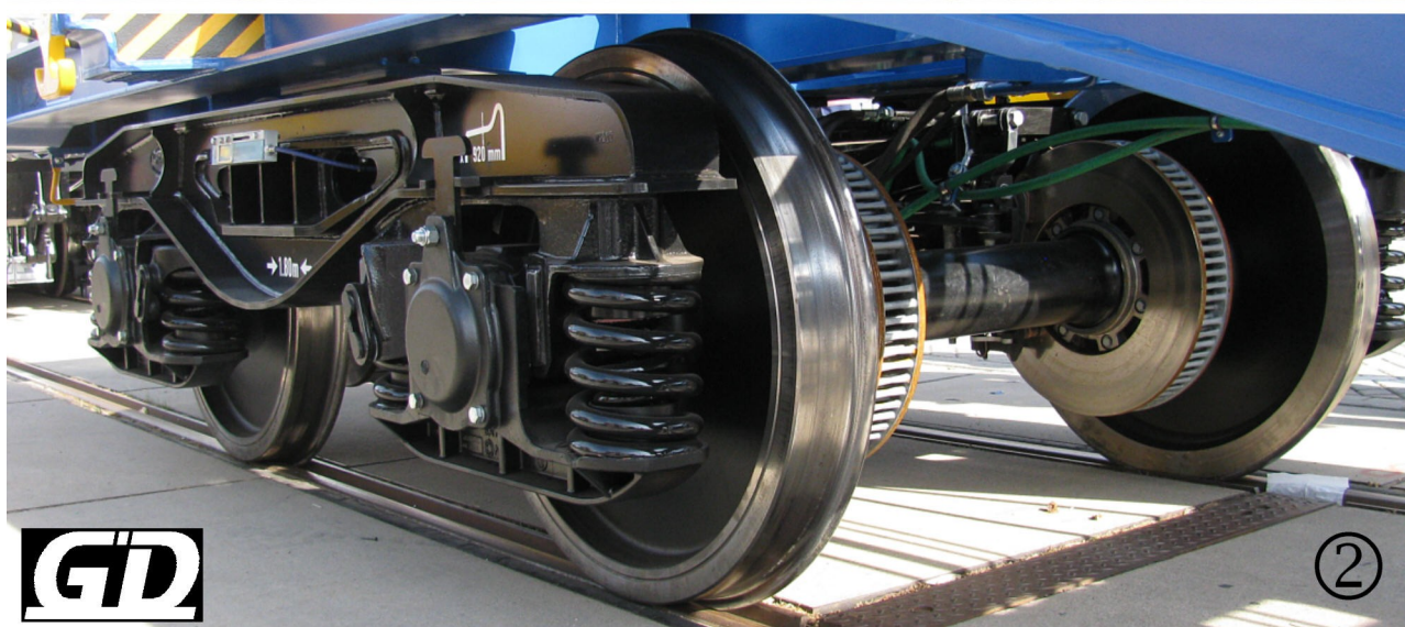
Güterwagen-Drehgestelle Legios Y 25Lssi(f)-D, gesehen auf den Freigelände und unter 33 TEN 54 CZ-LGSL 4594 001-8 Sgmmnss
