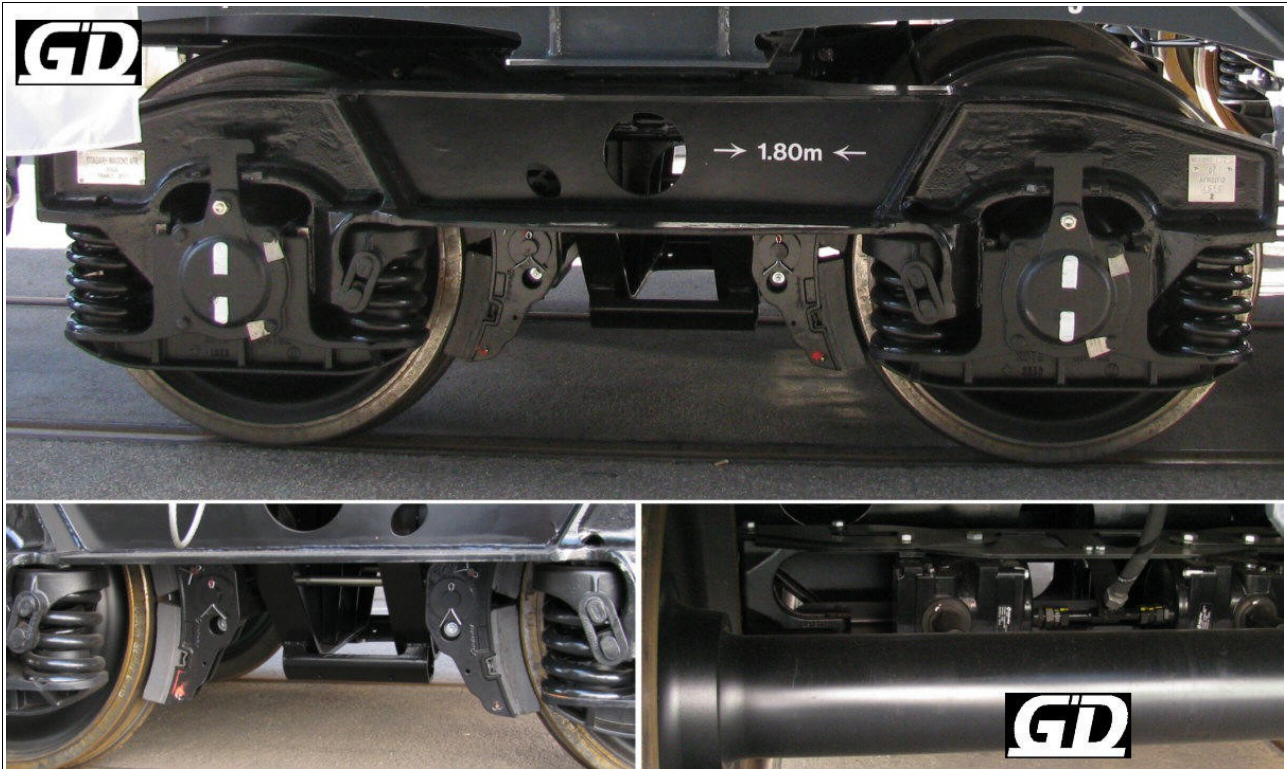
Güterwagen-Drehgestell AFR22Fi2 unter 33 TEN 87 F-ERS 0764 817-0 Tagnpps (1), gesehen auf dem Freigelände Freight Car Bogie AFR22Fi2 with 33 TEN 87 F-ERS 0764 817-0 Tagnpps (1), seen at outdoor display
